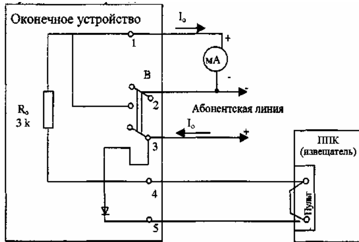
Рисунок П1.1 - Схема измерения тока системы "Центр-М"
