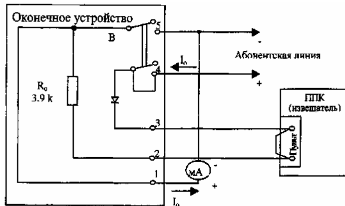
Рисунок П1.3 - Схема измерения тока систем "Нева-10М" и "Нева-10"
