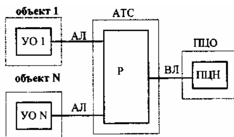
Рисунок 5.1 - Структура СПИ
