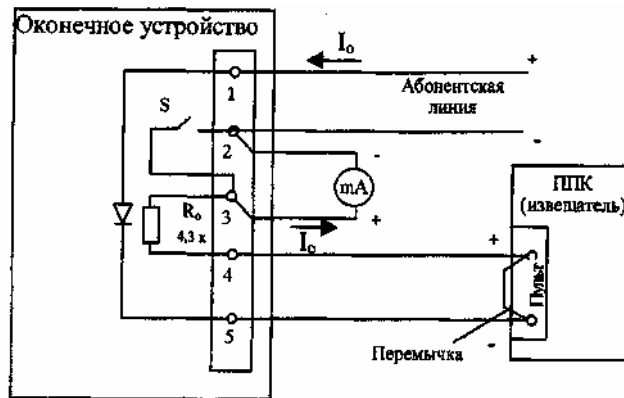
Рисунок П1.2 - Схема измерения тока системы "Центр-КМ"
