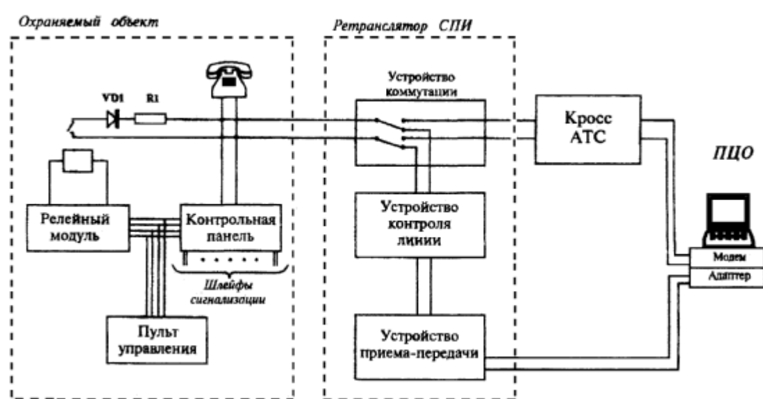
Рисунок 1 - Реализация КСЦО с использованием релейного модуля
