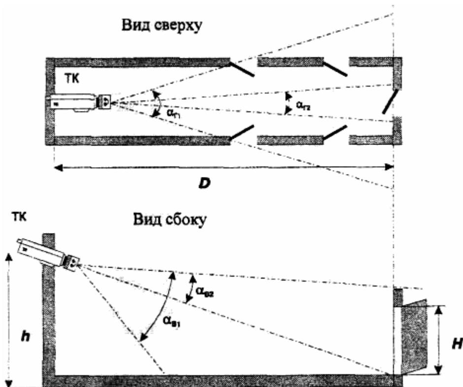
Рисунок 5 - Схемы охраны коридора
