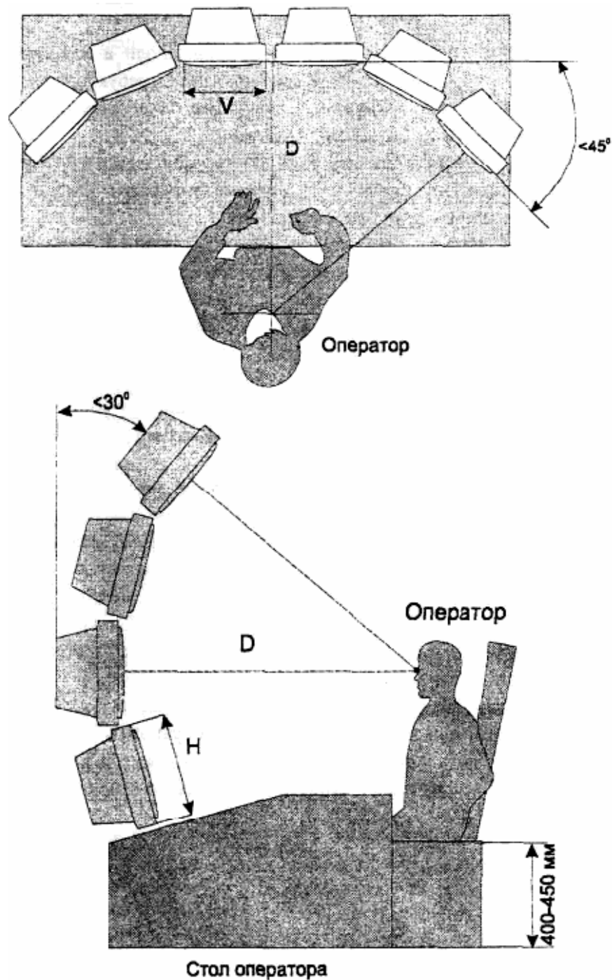
Рисунок 3 - Схема рабочего места оператора
