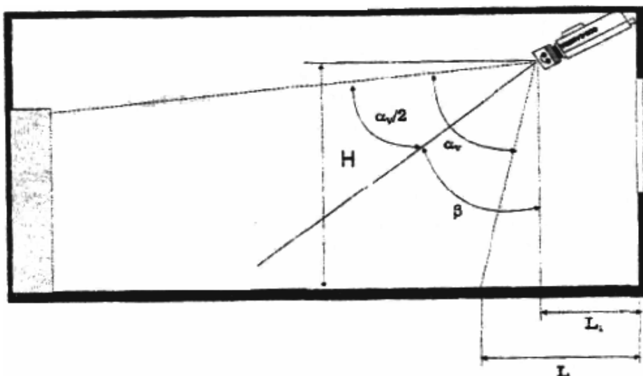
Рисунок 2 - "Мертвая" зона ТК (вид сбоку)
