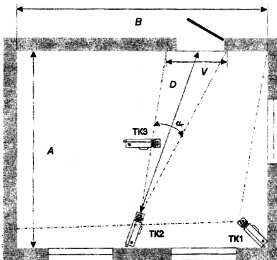
Рисунок 4 - Схема охраны помещения
