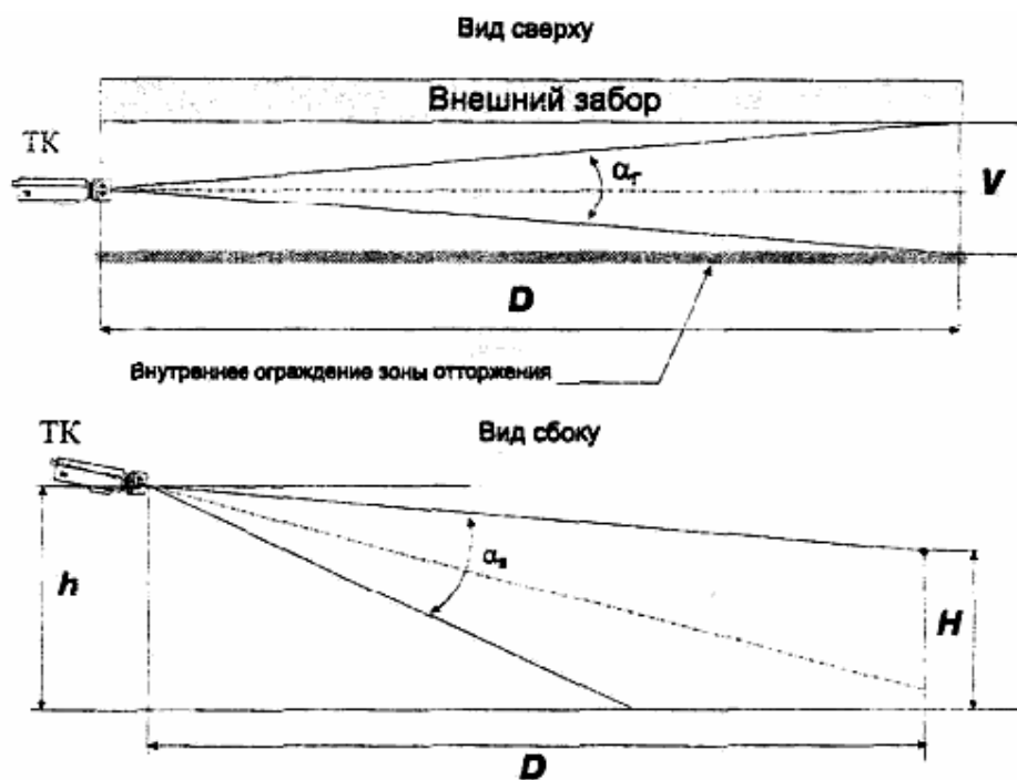
Рисунок 7 - Схемы охраны периметра
