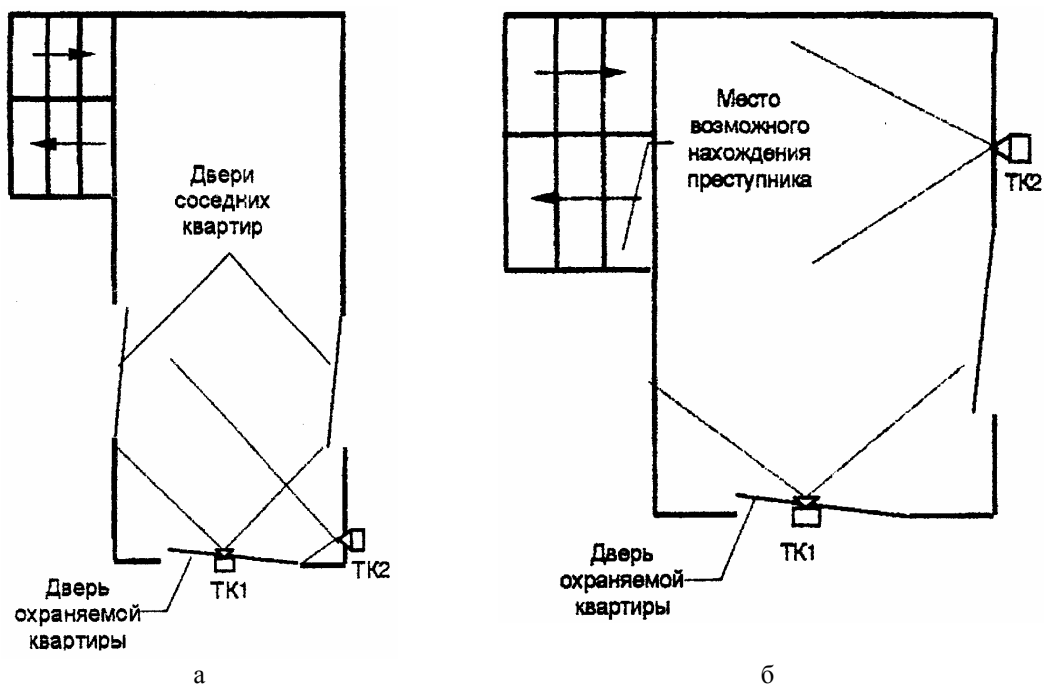
Рисунок 17 - Обзор пространства с помощью дополнительной ТК: а - сбоку от входной двери; б - лестничного пролета
