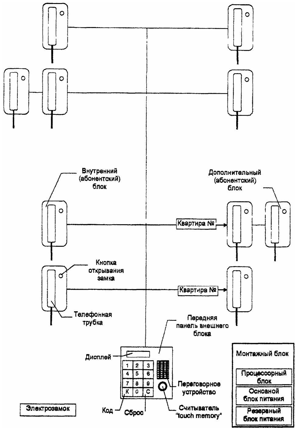
Рисунок 12 - Типовая конфигурация одноуровневого подъездного аудиодомофона
