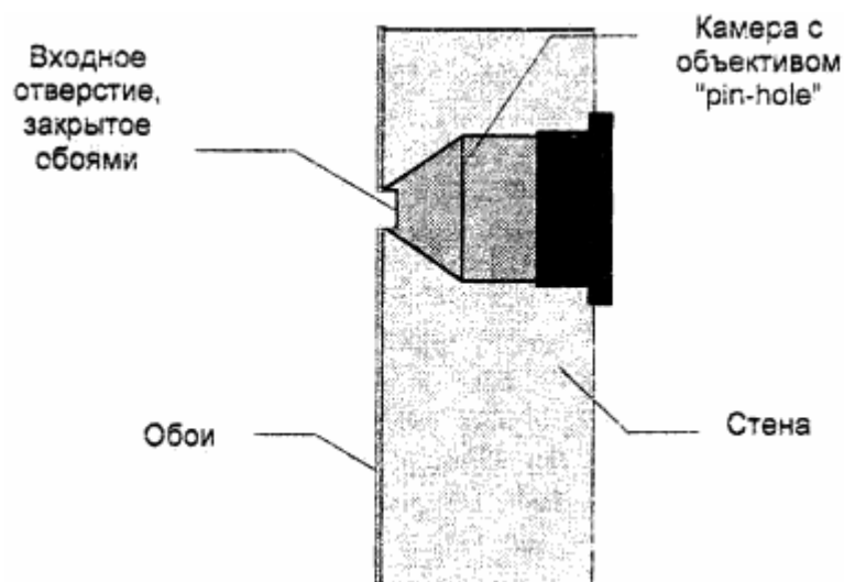
Рисунок 16 - Вариант установки видеоглазка в стене под обоями
