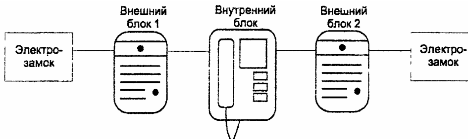
Рисунок 11 - Схема домофона из двух камер и одного монитора
