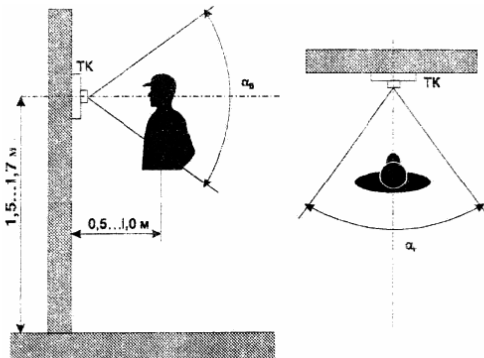
Рисунок 14 - Углы обзора камеры видеодомофона по вертикали ( \alpha_B ) и горизонтали ( \alpha_r )
