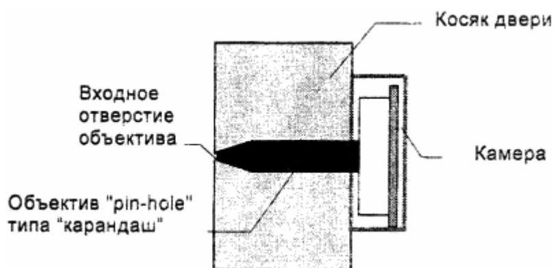
Рисунок 15 - Вариант установки видеоглазка в дверном косяке
