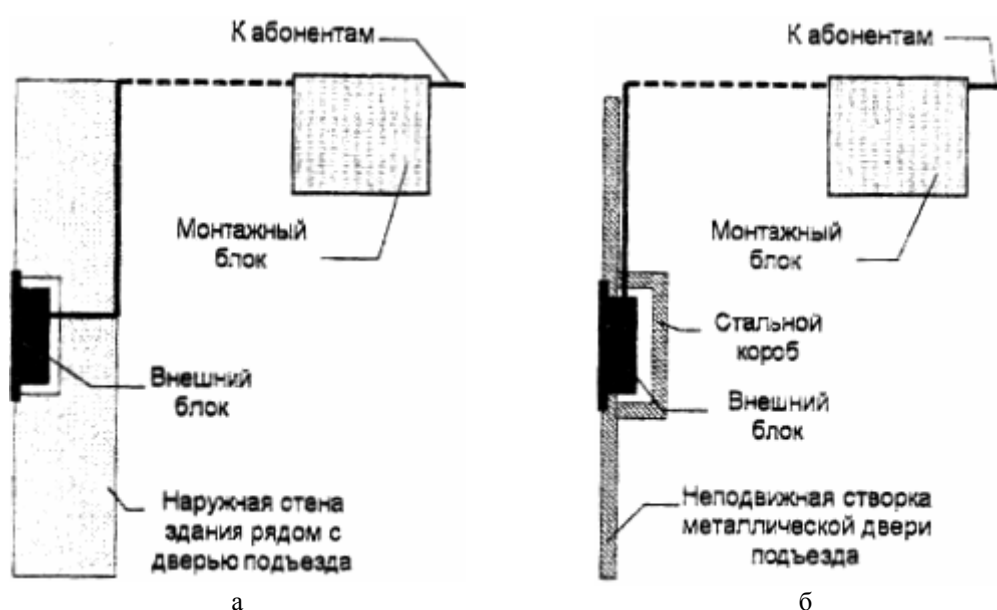
Рисунок 18 - Варианты монтажа блоков подъездного домофона: а - с установкой внешнего блока на стене здания; б - с установкой внешнего блока на металлической двери
