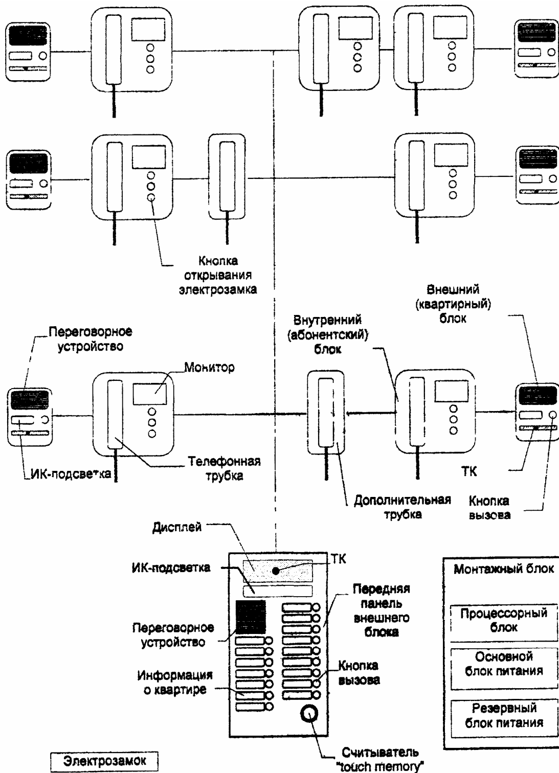
Рисунок 13 - Типовая конфигурация двухуровневого подъездного видеодомофона
