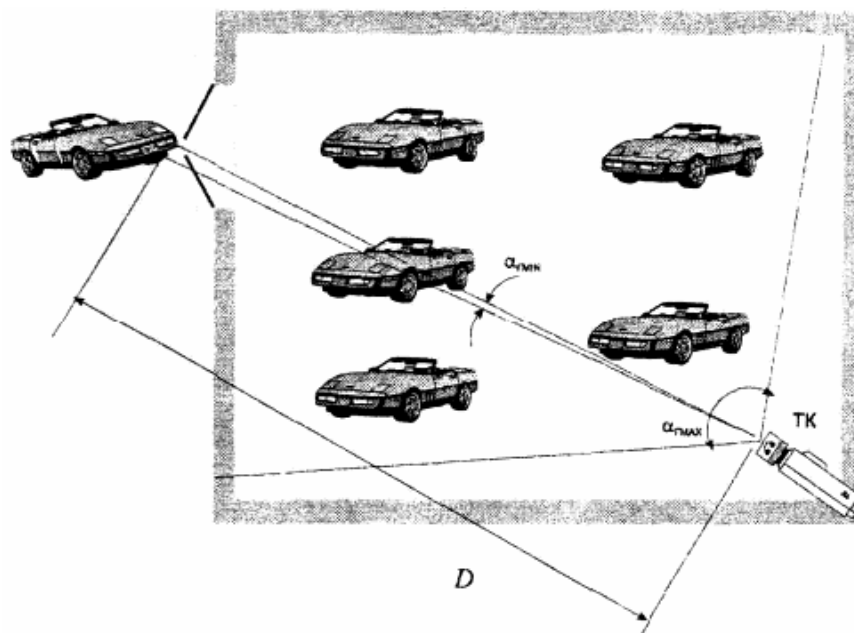
Рисунок 8 - Схема охраны стоянки автомобилей
