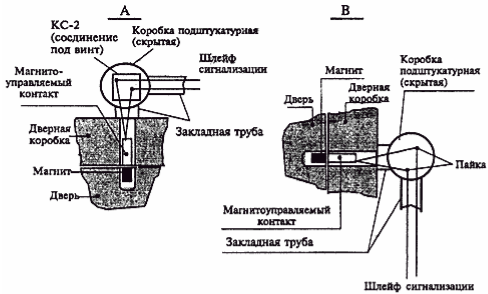
Рисунок 1 - Варианты установки магнитоcontactных извещателей на дверь
