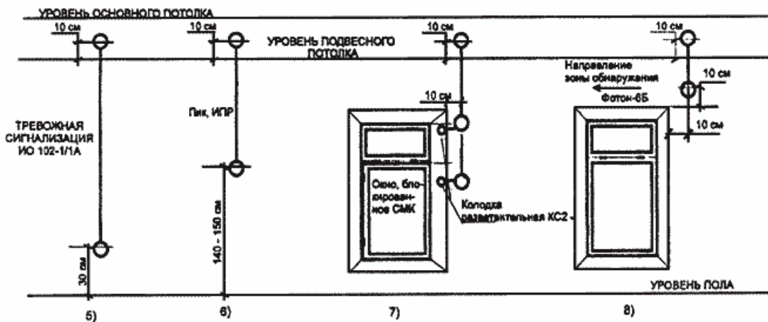
Рисунок 4 - Варианты расположения закладных для ТС ОПС в помещениях объекта
