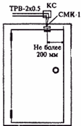
I Вариант установки (открытая установка)
