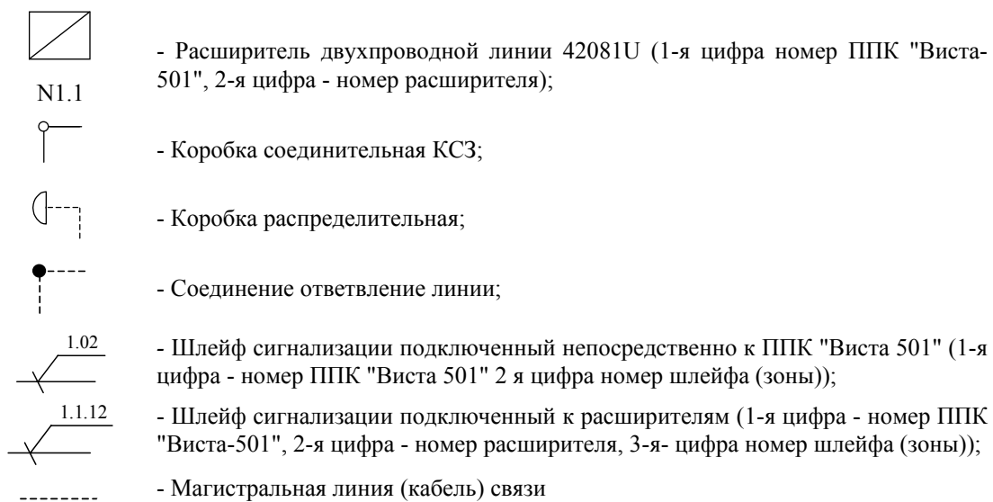
Рисунок 6 - Вариант выполнения схемы плана сети охранной сигнализации на базе ППК "Виста-501"
