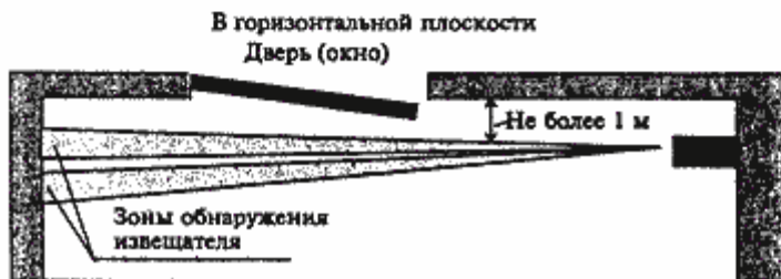
Рисунок 2 - Вариант блокировки двери (окна) на открывание и проникновение. (Размещение и схема подключения извещателей)
