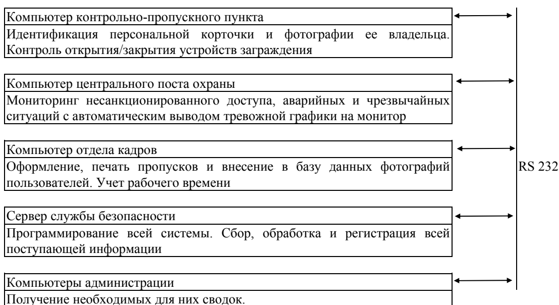
Рисунок 7 - Примерное размещение компьютеров СКУД, объединенных в сеть, на объекте
