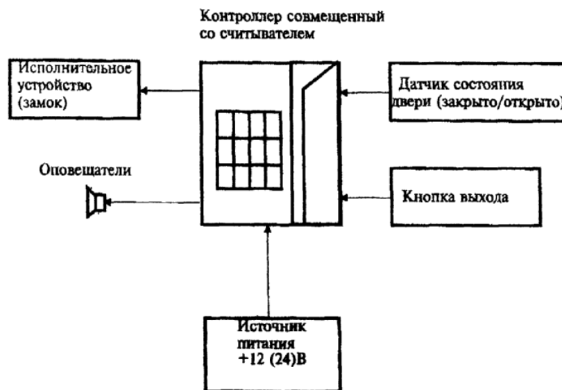
Рисунок 1 - Оборудование СКУД помещения с одной дверью
