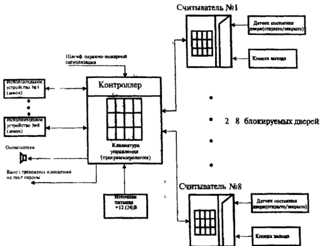
Рисунок 2 - Оборудование СКУД объекта с несколькими дверями
