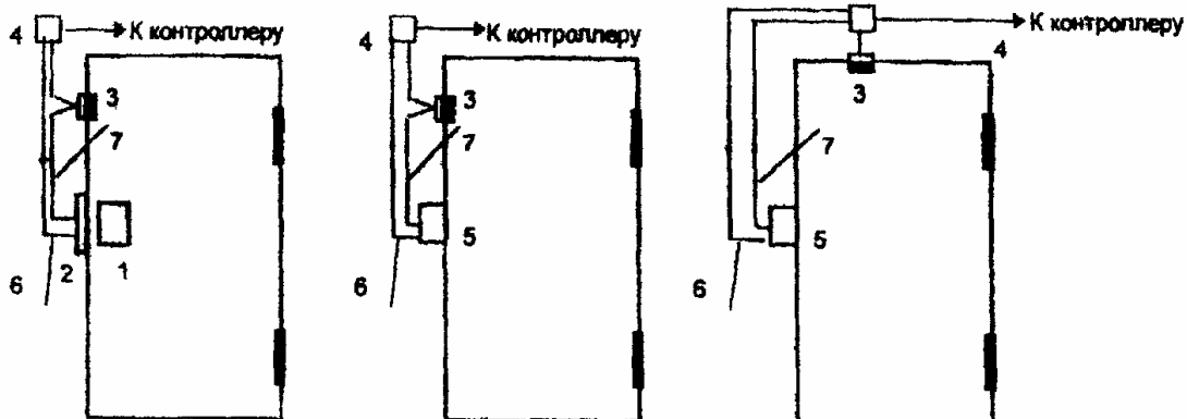
Рисунок 8 - Варианты размещения считывателей
