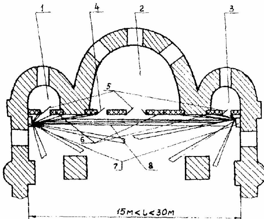
Рис. 1 - Вариант блокировки иконостасов алтарей, размещенных в ряд 1 - помещение алтаря северного предела; 2 - помещение центрального алтаря; 3 - помещение алтаря южного предела; 4 - боковая входная дверь в алтарные помещения; 5 - царские ворота иконостасов; 6 - иконостасы алтарей; 7 - извещатели "Фотон-6" ("Фотон-7"); 8 - элементарные зоны обнаружения извещателями.
