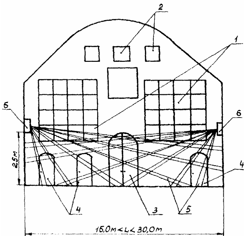
Рис. 2 - Зона блокировки извещателями "Фотон-6" ("Фотон-7") иконостасов алтарей
