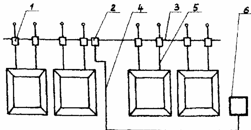
Рис. 6 - Вариант блокировки извещателем "Гюрза-050" нескольких икон.
