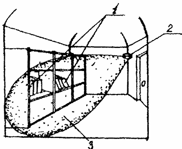
Рис. 4 - Вариант блокировки церковных ценностей в алтарном помещении извещателем "Волна-М" 1 - стеллажи с иконами, 2 - извещатель "Волна-М", 3 - зона обнаружения извещателя.
