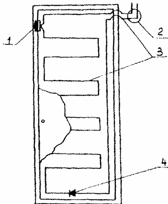
Рис. 11 - Вариант блокировки двери проводом на "пролом"
