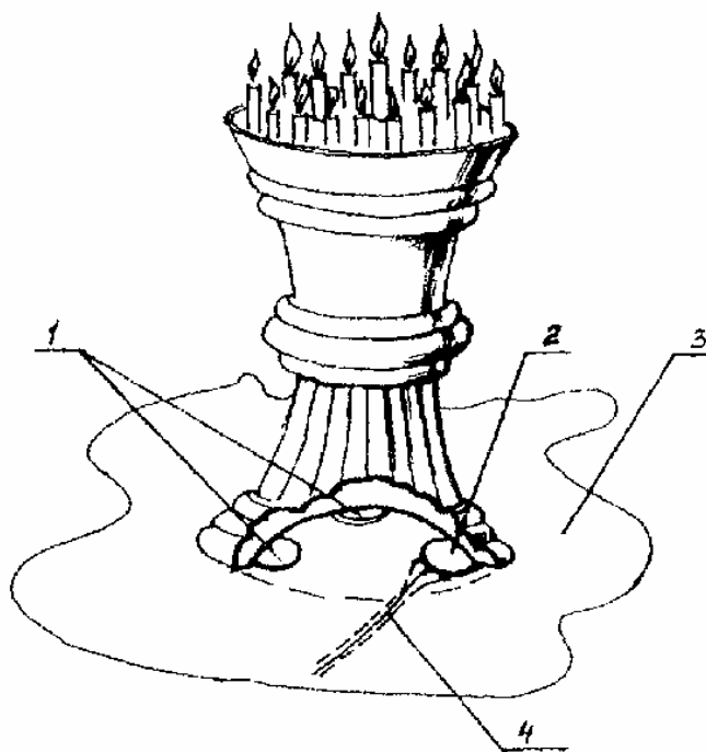
Рис. 8 - Вариант блокировки напольного подсвечника извещателем "Гюрза-050"
