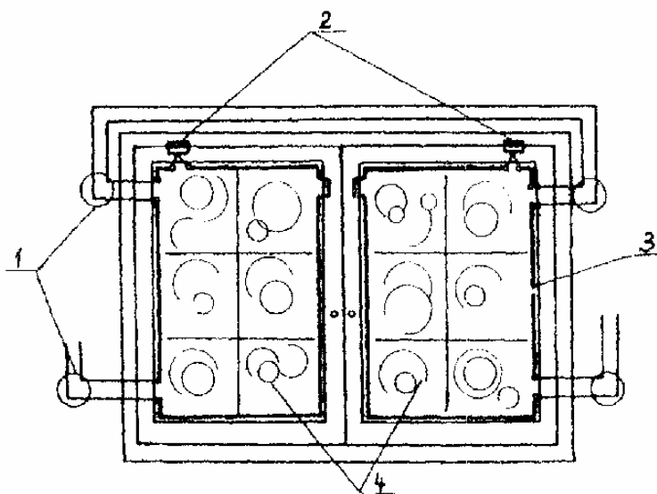
Рис 9. Вариант блокировки на разбитие стекла дверцы киота с использованием алюминиевой фольги
