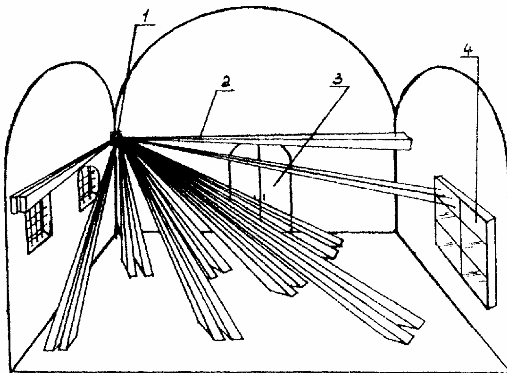
Рис. 3 - Вариант блокировки иконостаса алтаря извещателем "Фотон-4" 1 - извещатель "Фотон-4"; 2 - элементарные зоны обнаружения извещателя; 3 - царские ворота; 4 - настенный киот. Такой вариант обеспечивает надежную защиту не только иконостаса, но и объема всего помещения вместе с другими церковными предметами и предотвращает проникновение в охраняемое помещение через пол, потолок, стены и окна. При блокировке церковных помещений, объем которых заполнен большим количеством предметов церковной утвари, а также помещений (алтарные помещения, хранилища икон, ризницы и т.п.), имеющих легкие деревянные перегородки, целесообразно использовать радиоволновые извещатели. Это позволит надежно защитить пространство перед предметами (иконами, перегородками и т.п.) и за ними. На рис. 4 приведен вариант блокировки радиоволновым извещателем "Волна-М"
